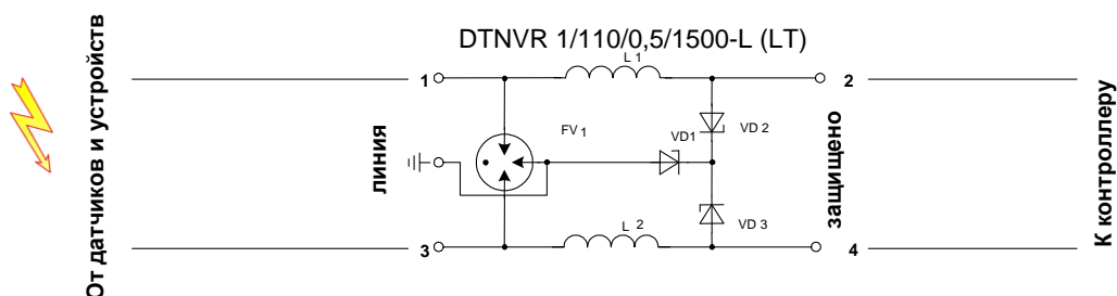
Пример типовой защиты линии
