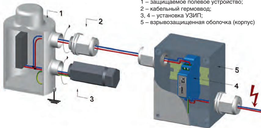
▲ Монтаж устройства DTNVR во взрывоопасной зоне
