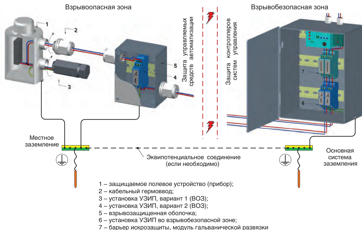
▲ Применение УЗИП DTNVR и ГИК: комплексная защита средств автоматизации
