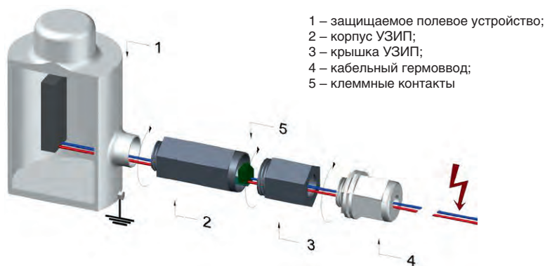
▲ Монтаж УЗИП ГИК 6/х во взрывоопасной зоне: последовательное включение
