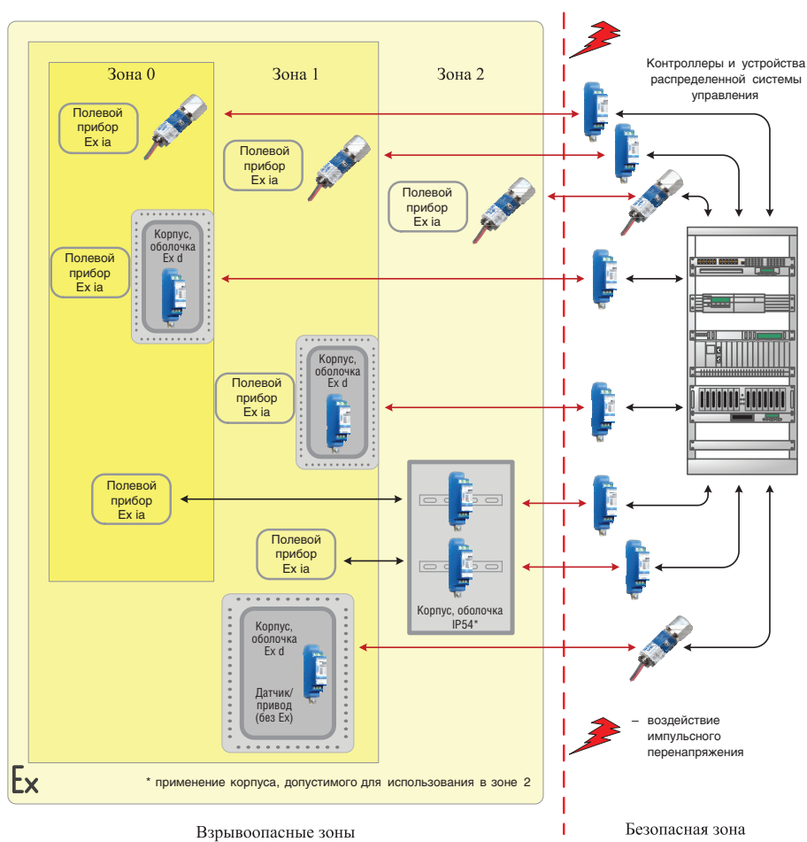
▲ Примеры размещения УЗИП для ВОЗ в цепях автоматизации
