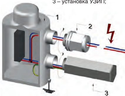
▲ Способ монтажа УЗИП серии ГИК 24/3: параллельная прокладка
